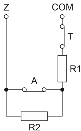
Obr. 4. Číslovanie vyvažovacích rezistorov. T – sabotáž. A – alarm. V prípade konfigurácie EOL je hodnota rezistora sumou hodnôt naprogramovaných pre rezistory R1 a R2.
