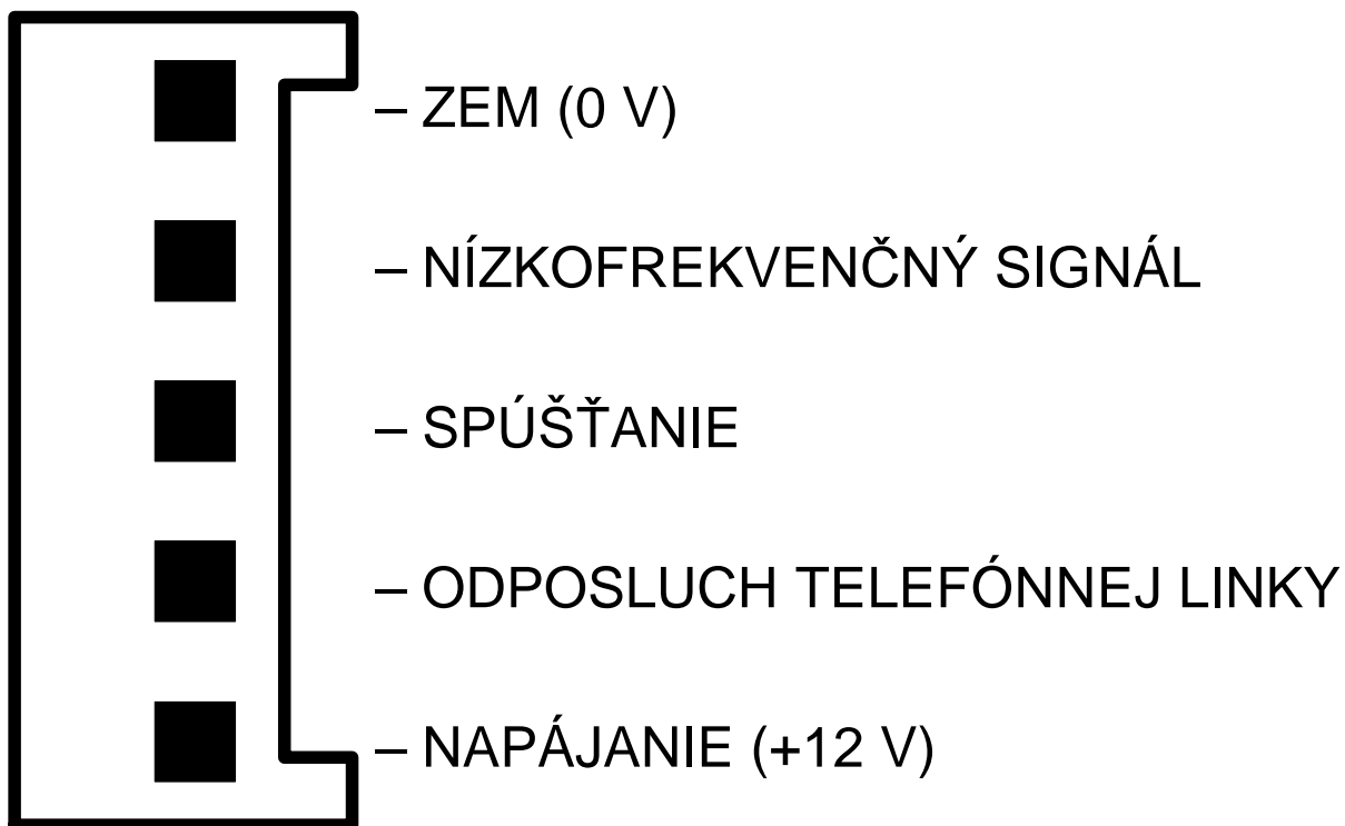
Obr. 1. Rozloženie signálov na kontaktoch konektora hlasového modulu SM-2.
