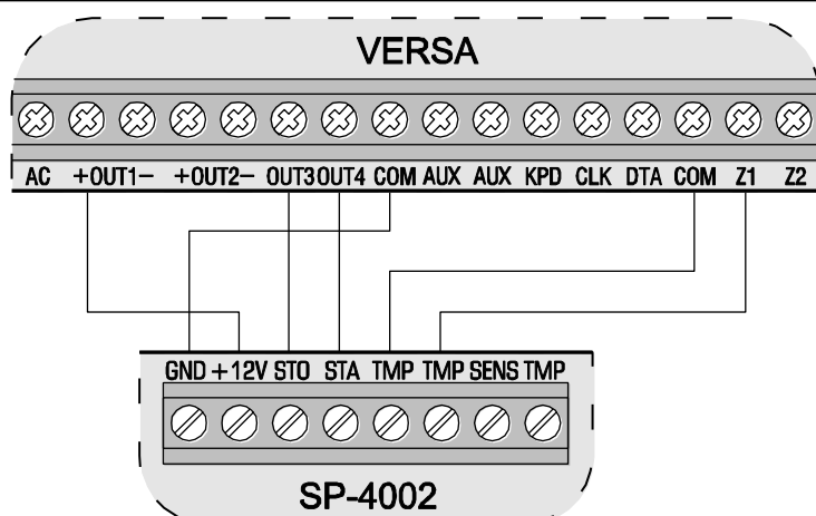
Obr. 29. Spôsob pripojenia sirény s vlastným napájaním na ústredňu (na príklade SP-4002). Pre vstupy OUT3 a OUT4 treba naprogramovať opačnú polaritu. Jumpy PLO a PLA na siréne musia byť zložené (signalizácia spúšťaná odpojením zeme napájania).
