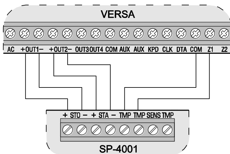
Obr. 28. Spôsob pripojenia sirény bez vlastného napájania na ústredňu (na príklade SP-4001).
