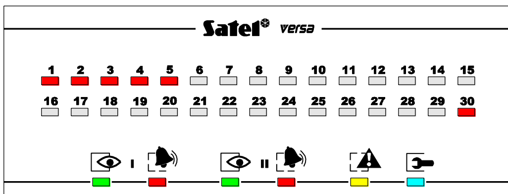
Obr. 9. Programovanie adresy LED klávesnice. LED-ky označené číslami 1 až 5 a 30 sa používajú na zobrazenie adresy (30 – pre adresu 0). LED-ka, ktorá zodpovedá aktuálnej adrese rýchlo blika a ostatné svietia.
